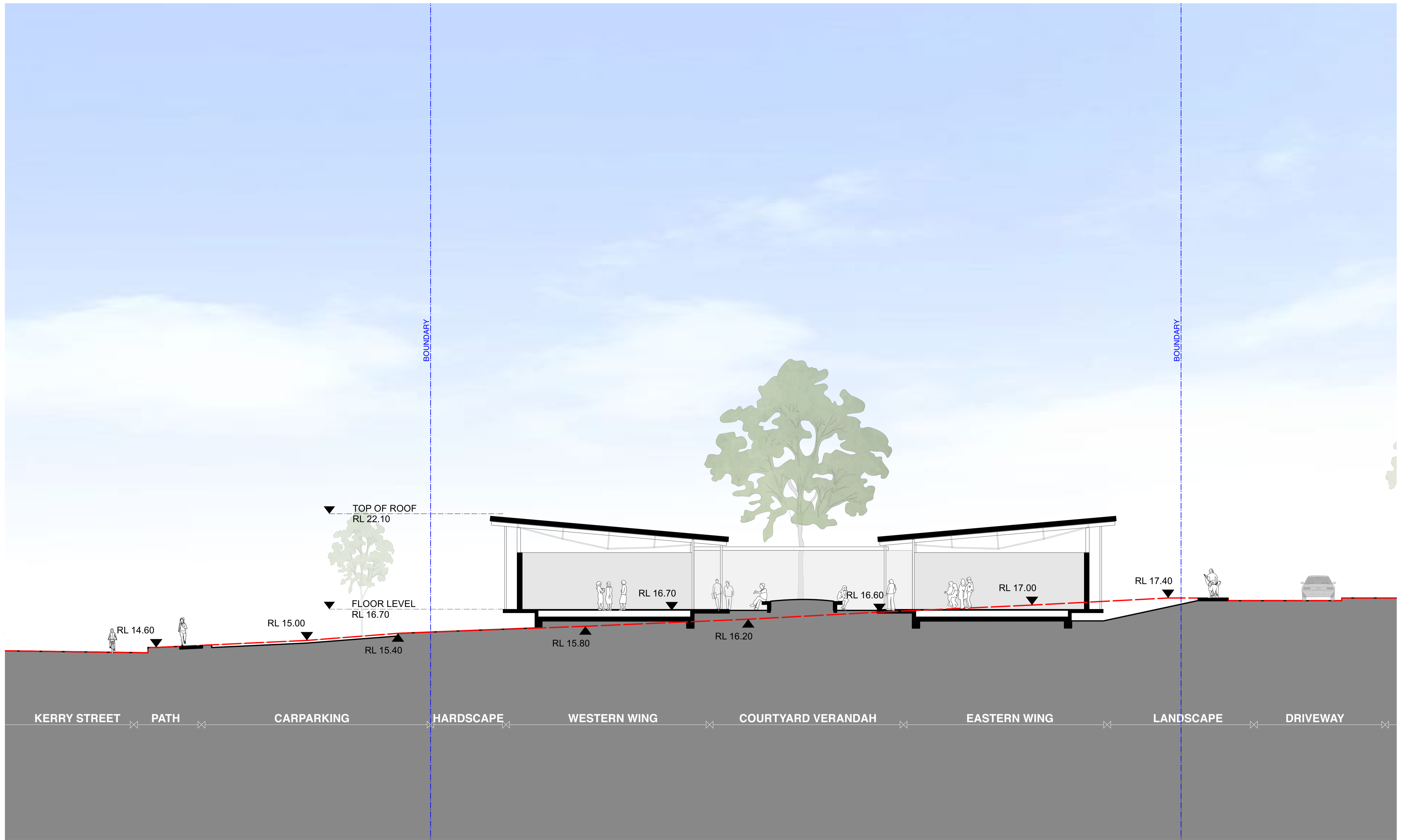
Section 1 | Scale 1 : 100
