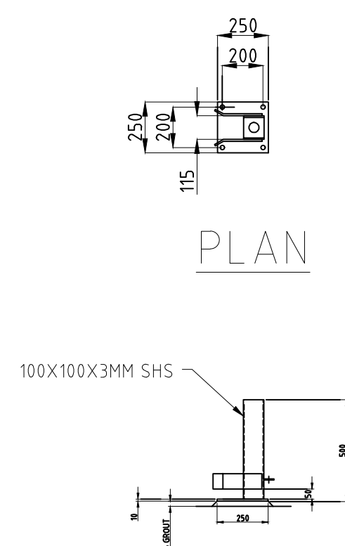
END ELEVATION
