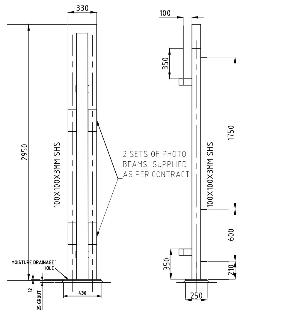
ELEVATION
