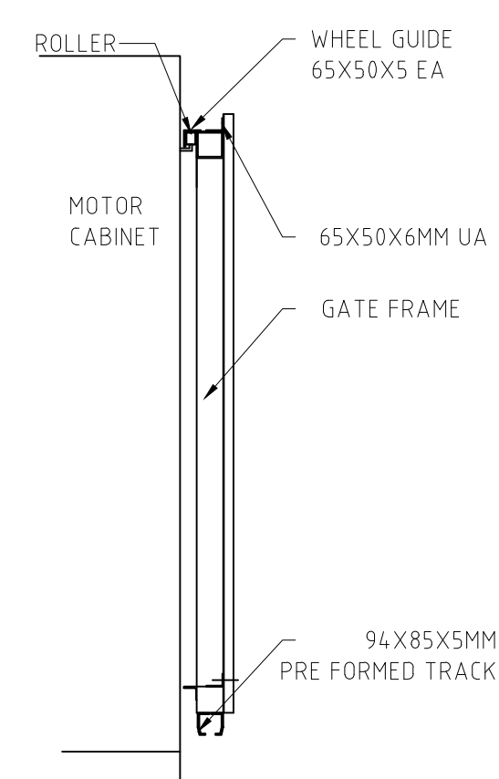
END ELEVATION
